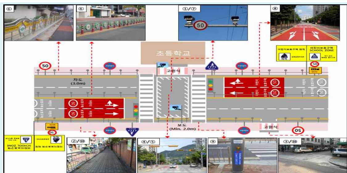
[그림 2] 어린이 보호구역 정비 표준모델(간선도로 C타입)
